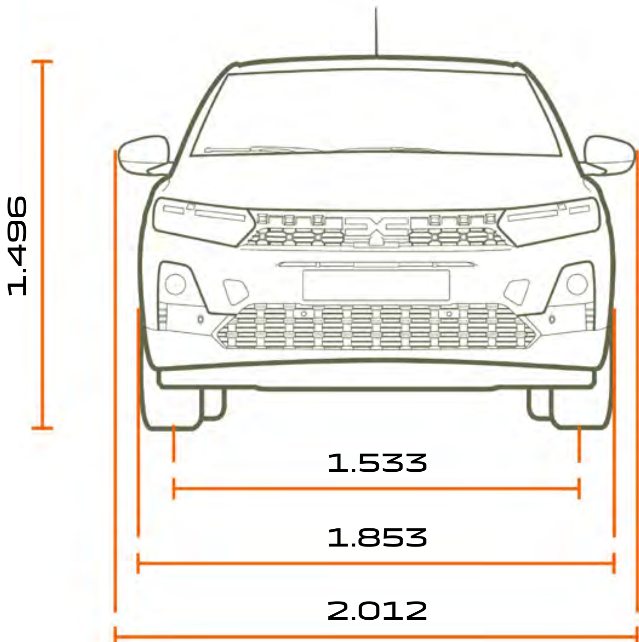
FRONTANSICHT
