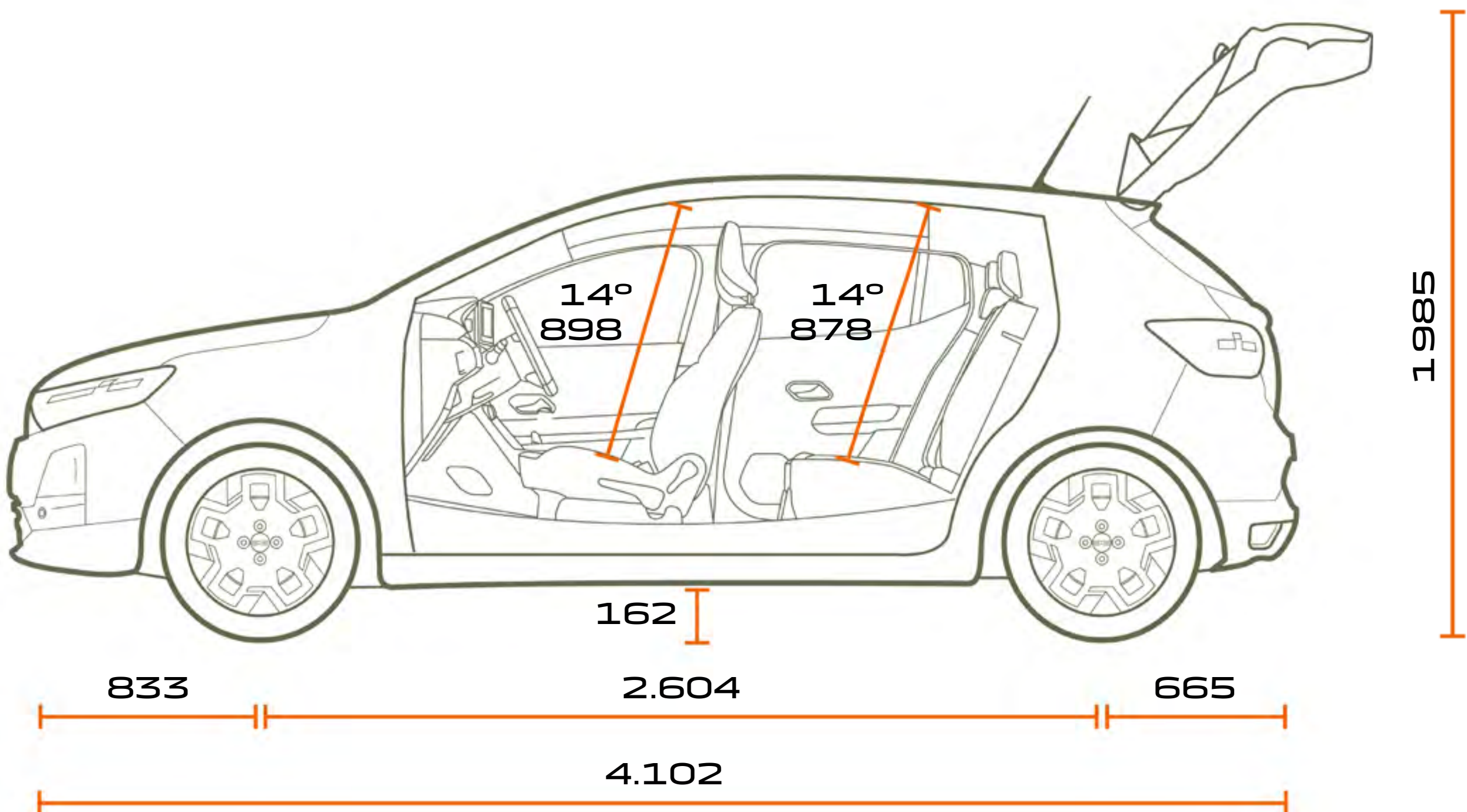
SEITENANSICHT
