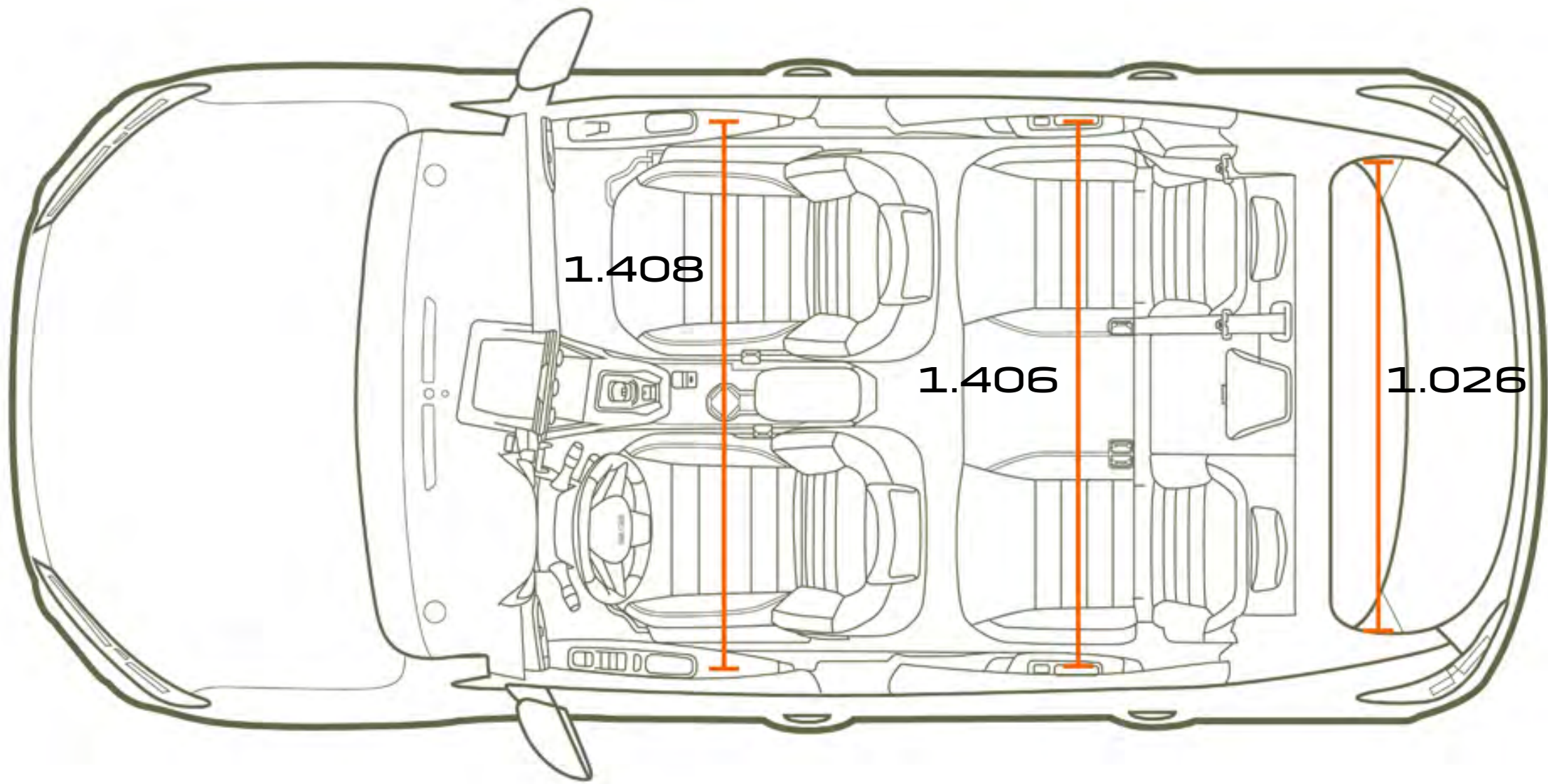
ANSICHT VON OBEN
