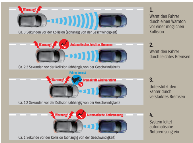
Radargestützte aktive Bremsunterstützung (RBS) 1
